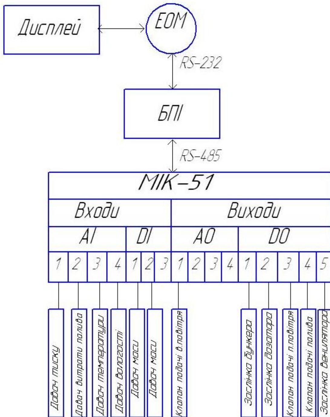
Рисунок 3. Структура системи управління
