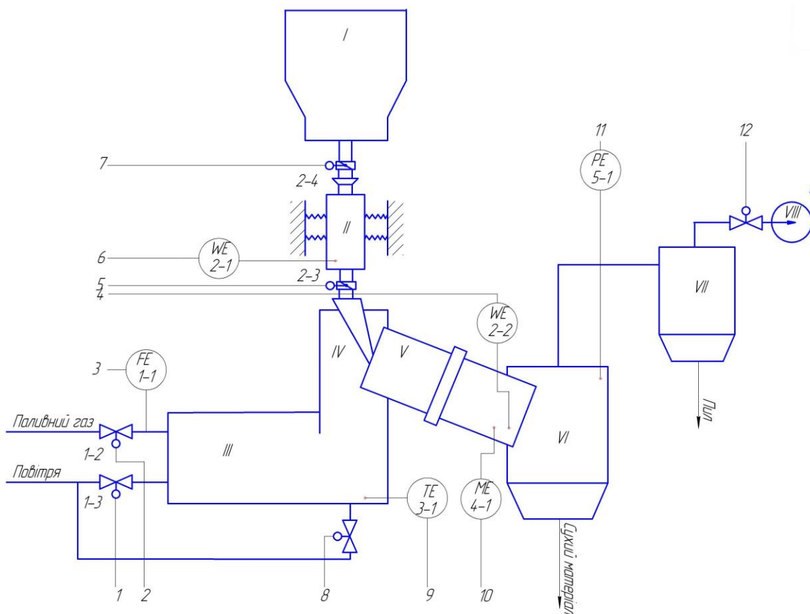
Рисунок 2. Функціональна схема автоматизації процесу сушіння в барабанній сушарці
